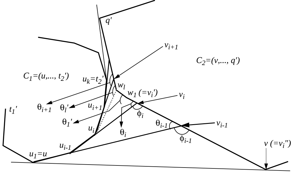
Figure 12: Lemma 11
