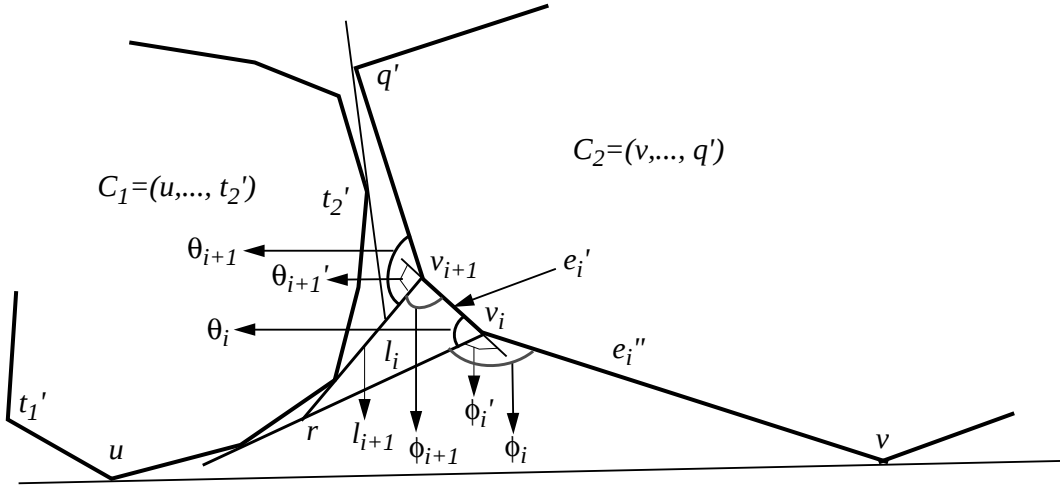
Figure 10: Lemma 8
