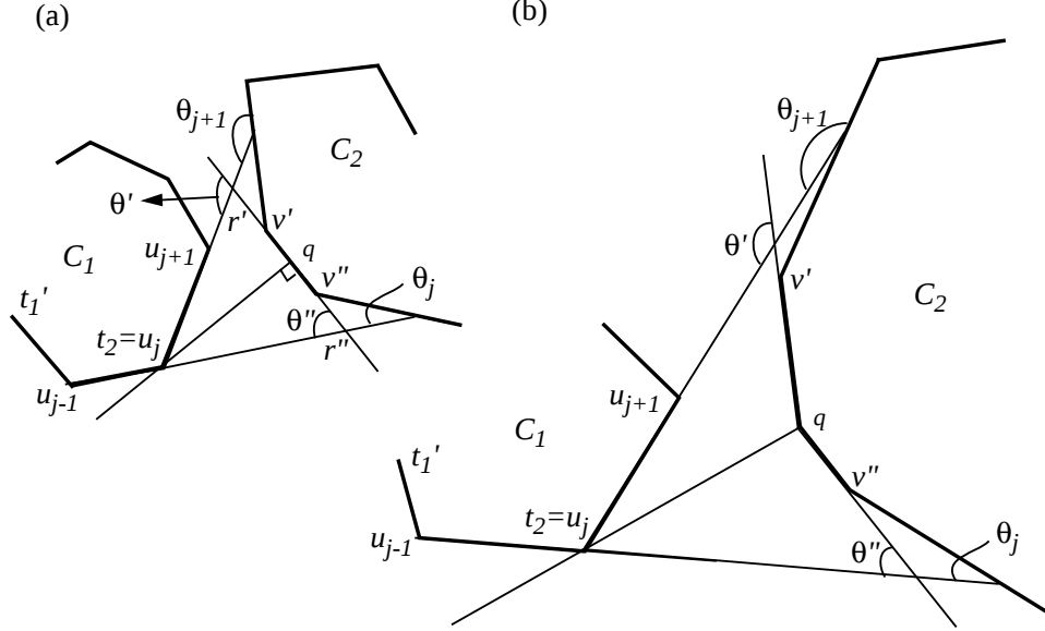
Figure 13: Lemma 12
